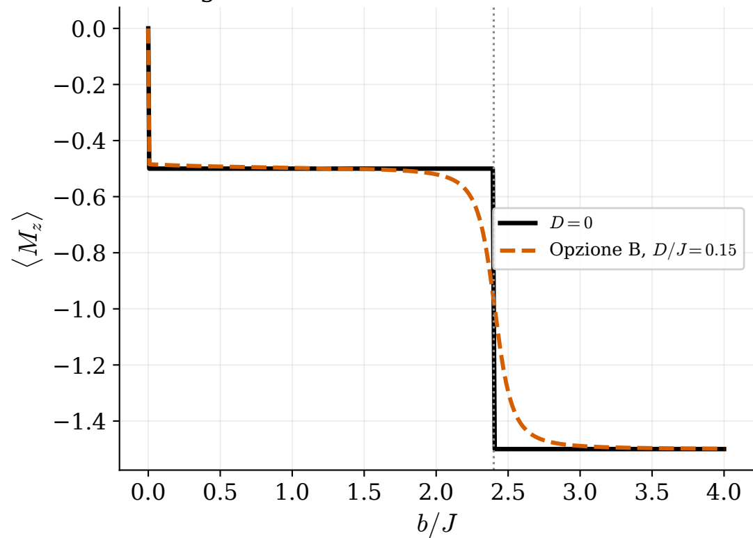
Magnetizzazione dello stato fondamentale
