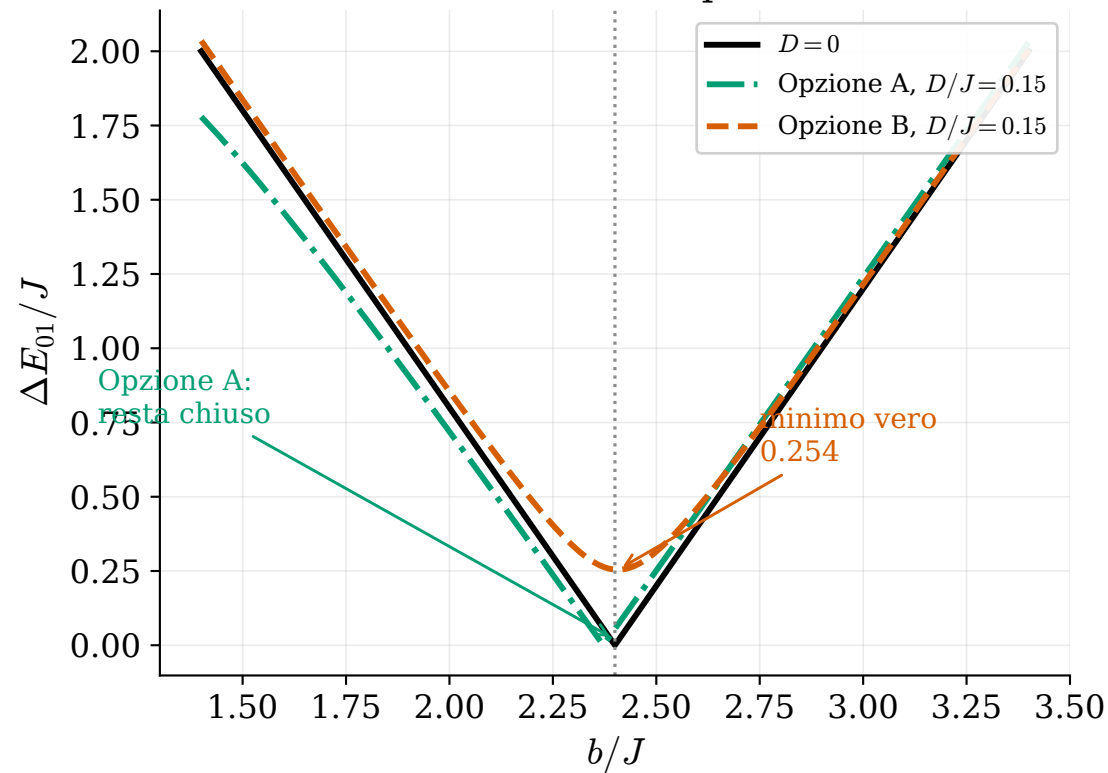
Distanza fondamentale-primò eccitato
